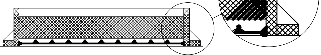
SECTION A-A
